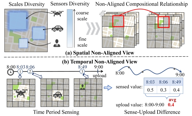
Fig. 1. The Spatiotemporal Non-Aligned Scenarios.
